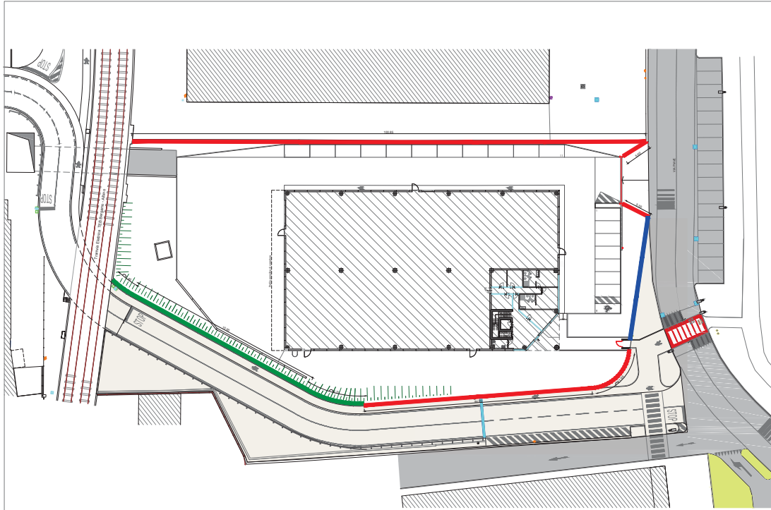
PLANIMETRIA GENERALE (scala 1:500)
