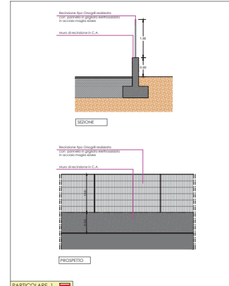
PARTICOLARE 1
