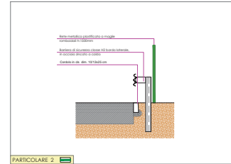
PARTICOLARE 2
