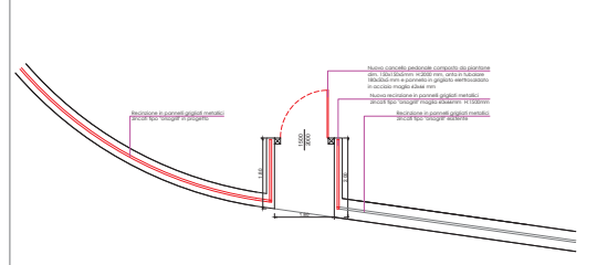
PIANTA ACCESSO PEDONALE IN PROGETTO (scala 1:50)
