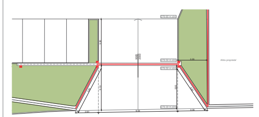
PIANTA ACCESSO CARRAILE IN PROGETTO (scala 1:100)
