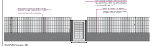
PARTICOLARE ACCESSO PEDONALE IN PROGETTO
