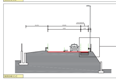
SEZIONE C-C
