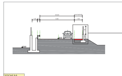
SEZIONE B-B
