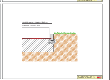
PARTICOLARE 5
