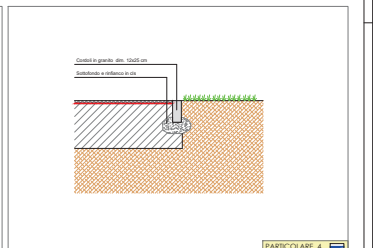
PARTICOLARE 4
