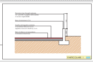
PARTICOLARE 1
