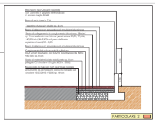
PARTICOLARE 2
