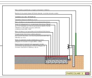
PARTICOLARE 3
