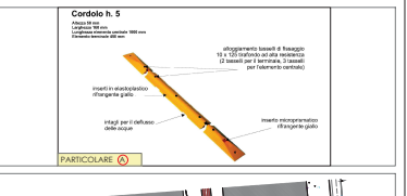
PARTICOLARE
