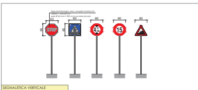
SEGNALETICA VERTICALE
