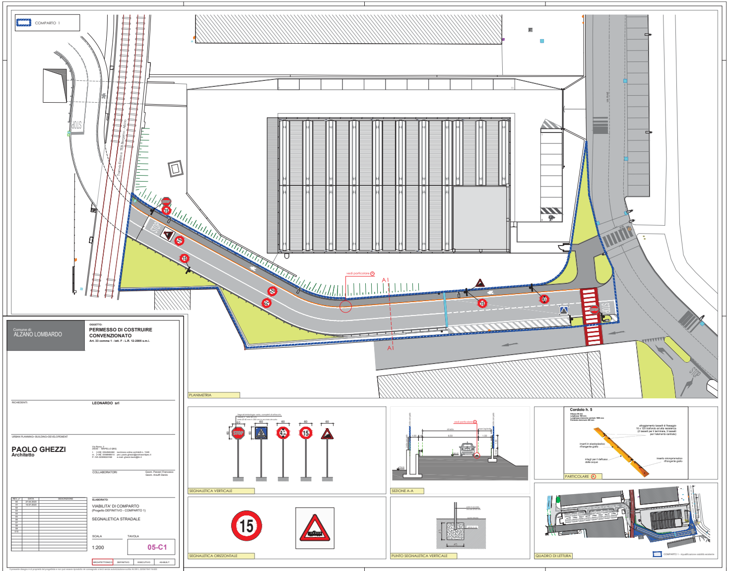
SEGNALETICA ORIZZONTALE
