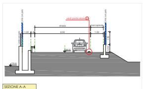
SEZIONE A-A
