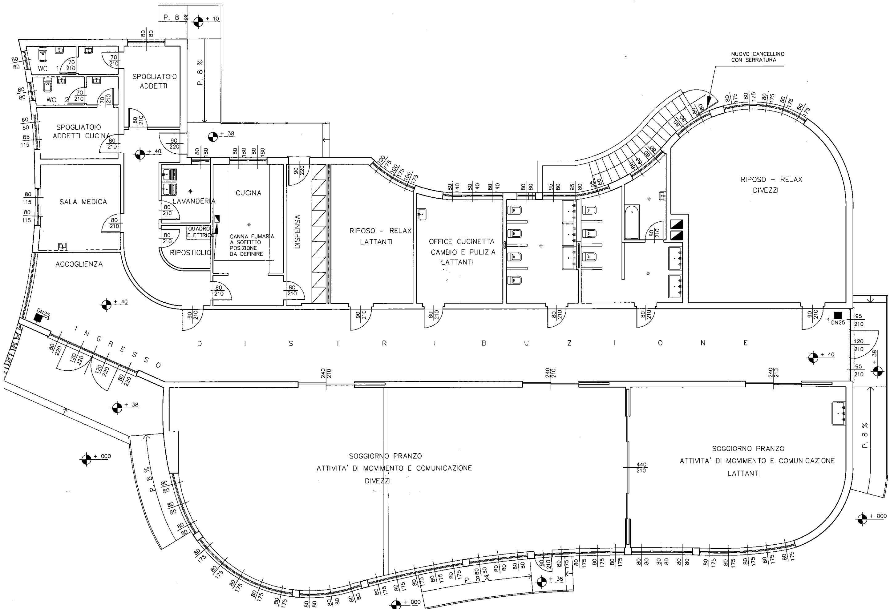
PLANIMETRIA GENERALE - SCALA 1:100
